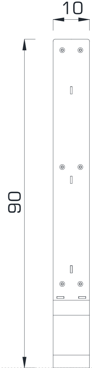
YAN GÖRÜNÜŞ / SIDE VIEW
