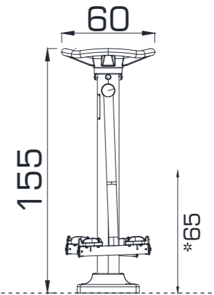
YAN GÖRÜNÜŞ / SIDE VIEW
