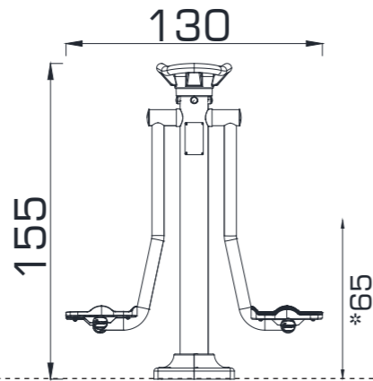
ÖN GÖRÜNÜŞ / FRONT VIEW
